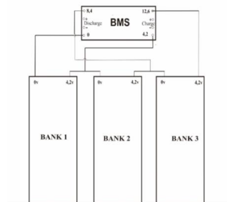
Gambar 2. Instalasi BMS Baterai
