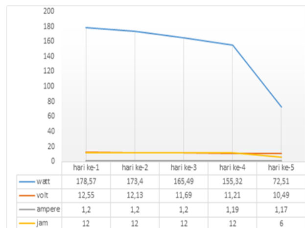
Gambar 4. Grafik pengujian dengan beban lampu DC
