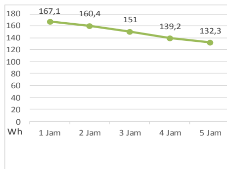
Gambar 5. grafik pemakaian multibeban
