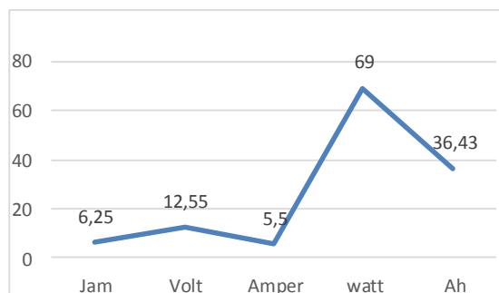
Gambar 3. grafik pengisian baterai pack
