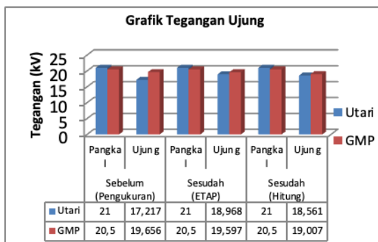
Gambar 3.3. Grafik Tegangan Ujung
