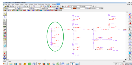
Gambar 2. Gambar Tegangan Ujung Penyulang GMP Sesudah Penambahan.
