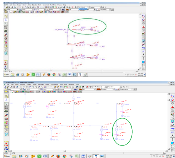
Gambar 1. Gambar Tegangan Ujung Penyulang Utari Sesudah Pengurangan.
