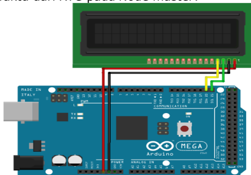
Gambar 5. Wiring Pengujian LCD pada Node master
