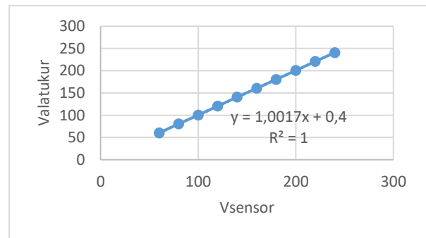
Gambar 14. Grafik Hubungan V Pembacaan Alat Ukur dan V Pembacaan Sensor Node 2
