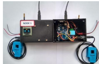
Gambar 2. Implementasi 2 Buah Node sensor
