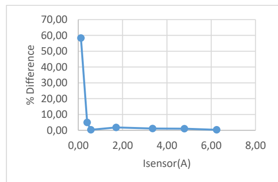
Gambar 17. Grafik Hubungan Persentase Differencedan I Pembacaan sensor Node 1
