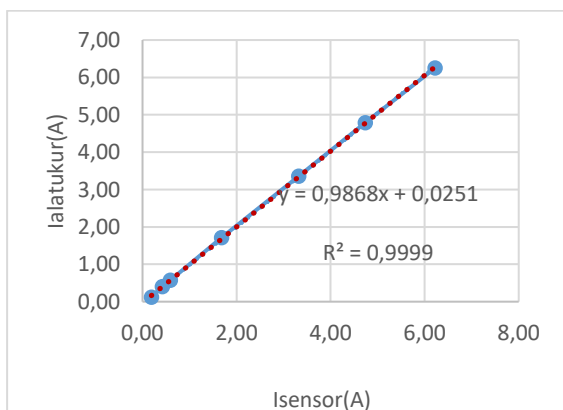
Gambar 18. Grafik Hubungan I Pembacaan alat ukur dan I Pembacaan sensor Node 2
