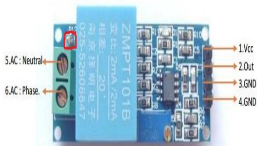
Gambar 10. Sensor Tegangan ZMPT101B
