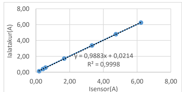
Gambar 16. Grafik Hubungan I Pembacaan alat ukur dan I Pembacaan sensor Node 1
