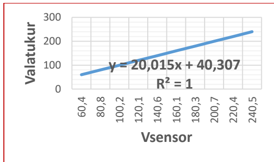
Gambar 12. Grafik Hubungan V Pembacaan Alat Ukur dan V Pembacaan Sensor Node 1
