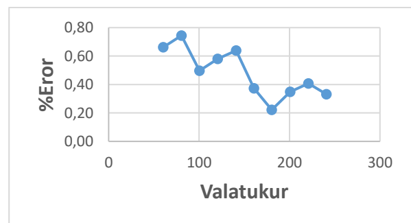
Gambar 15. Grafik Hubungan Persentase Difference dan V Pembacaan Alat Ukur Node 2
