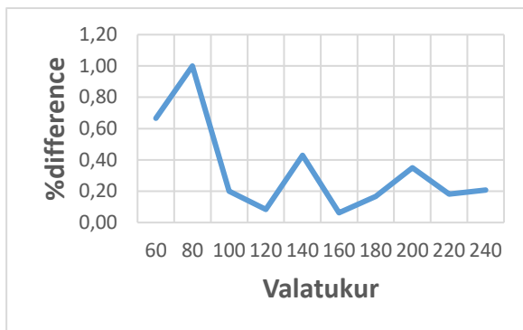
Gambar 13. Grafik Hubungan Persentase Difference dan V Pembacaan Alat Ukur Node 1
