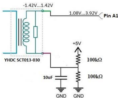
Gambar 15. Rangkaian dasar sensor arus YDHC SCT013-030 dengan pin A1 modul arduino
