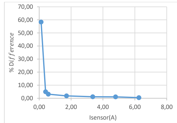
Gambar 19. Grafik Hubungan Persentase Difference dan I Pembacaan sensor Node 2
