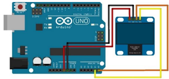
Gambar 7. Wiring pada Arduino UNO OLED Display 0,96"
