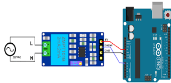
Gambar 11. Rangkaian dasar pengujian sensor ZMPT101B
