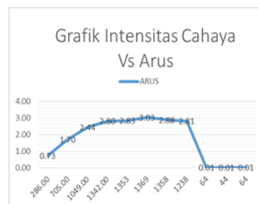
Gambar 8. Grafik Intensitas Cahaya Vs Arus pengukuran ke-3
