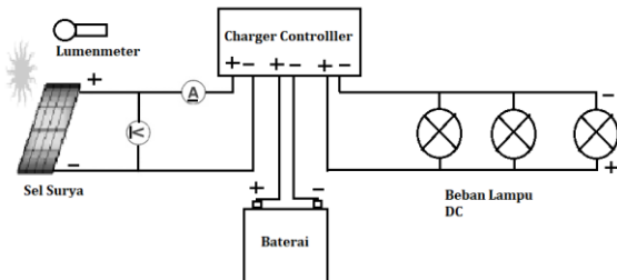
Gambar 5. Rangkaian Pengukuran SHS II
