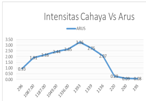
Gambar 11. Grafik Intensitas cahaya vs Arus pengukuran ke-4
