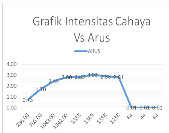
Gambar 9. Grafik Intensitas Cahaya Vs Arus pengukuran ke-3
