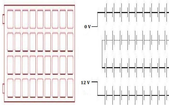
Gambar 2. Rangkaian Hubung Seri Solar Sel
