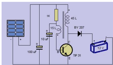
Gambar 1. Diagram Rangkaian
