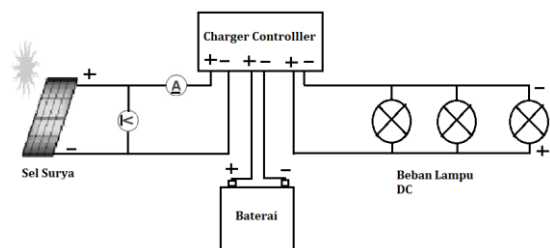
Gambar 4. Rangkaian Pengukuran SHS I
