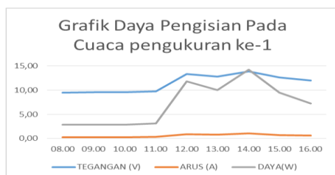
Gambar 6. Grafik Daya Pengisian ke-1
