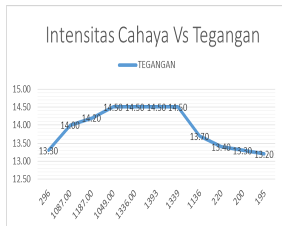
Grafik 10. Intensitas cahaya vs Tegangan Pengukuran ke-4
