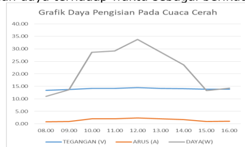
Grafik 7. Daya Pengisian Pada pengukuran ke-2
