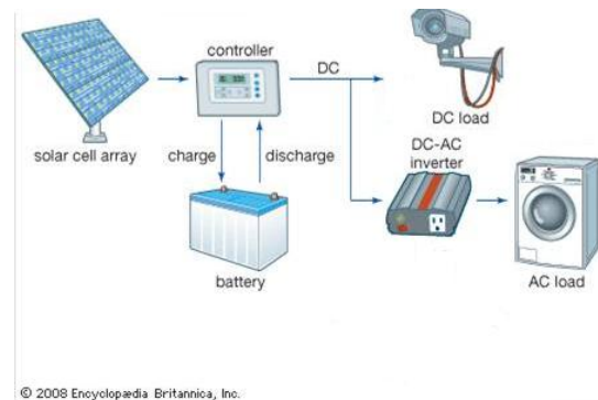
Gambar 5. Sistem PLTS
