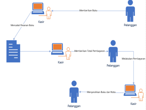
GAMBAR 2. AnalisisTransaksiPenjualan
