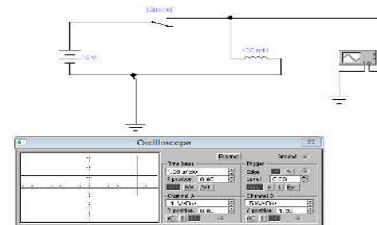
Gambar 3.2 Percobaan tanpa dioda dengan waktu 5 detik
