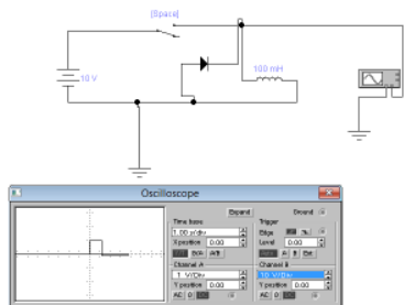
Gambar 3.3 Percobaan dengan dioda reverse bias dengan waktu 1 detik
