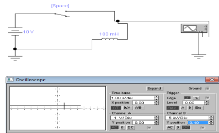
Gambar 3.1 Percobaan tanpa dioda dengan waktu 1 detik
