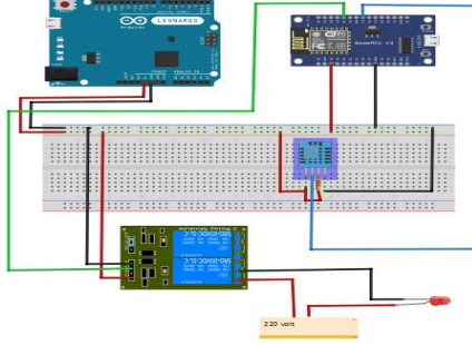
Gambar 4.1 Rangkaian NodeMCU ESP8266
