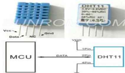
Gambar 2.3. Sensor Suhu dan Kelembaban DHT 11
