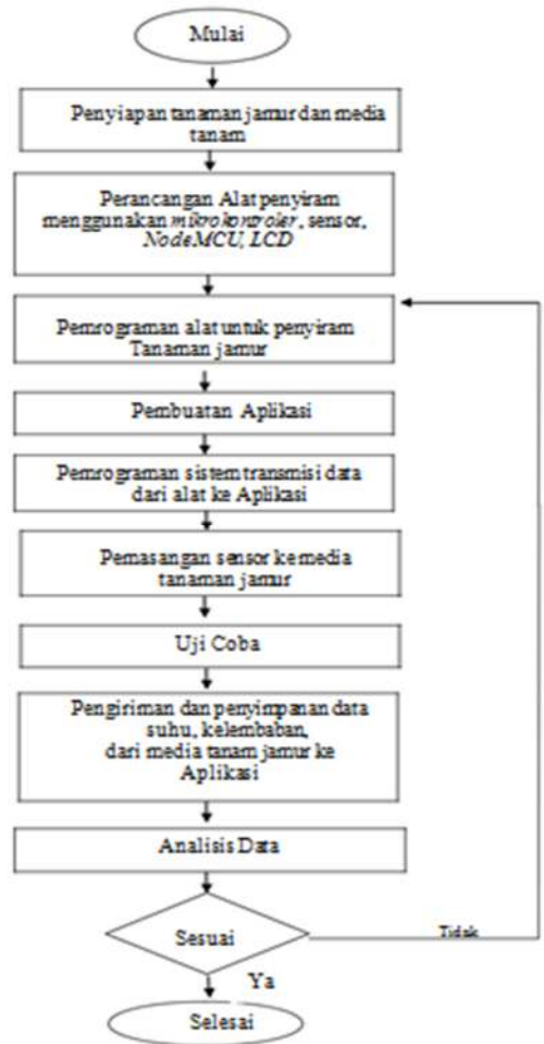
Gambar 3. Diagram Alir Metodologi
