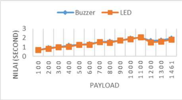
Gambar 4. grafik perbandingan Delay dengan output LED dan Buzzer
