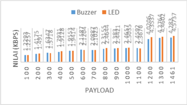
Gambar 2. grafik perbandingan Throughput dengan output LED dan Buzzer
