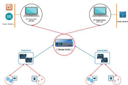
Gambar 1. Topologi pembuatan IoT dengan protokol CoAP
