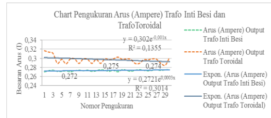
Gambar 21. Gabungan Grafik Pengukuran Arus (Ampere) Pada Trafo Inti Besi dan Trafo Toroidal menggunakan beban baterai kering (Lead Acid)
