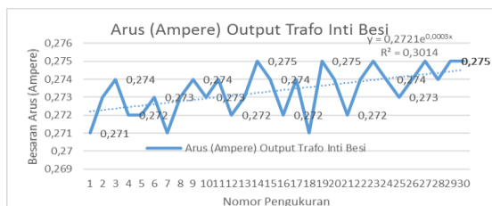
Gambar 19. Grafik Pengukuran Arus (Ampere) Pada Trafo Inti Besi menggunakan beban baterai kering (Lead Acid)
