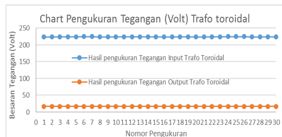
Gambar 15. Grafik Pengukuran Tegangan Trafo Toroidal menggunakan beban baterai kering ( Lead Acid )
