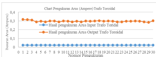
Gambar 16. Grafik Pengukuran Arus input dan output Trafo Toroidal menggunakan beban baterai kering (Lead Acid)
