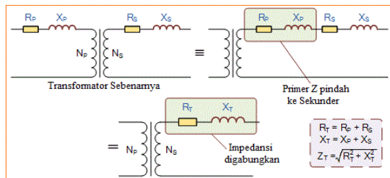
Gambar 4. Rangkaian Transformator dengan impedansi
