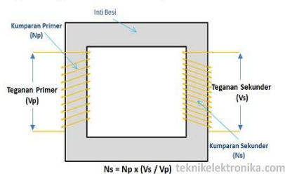
Gambar 7. Menghitung Jumlah Lilitan
