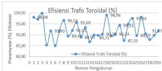
Gambar 18. Grafik Presentase (%) Efisiensi Trafo Toroidal
