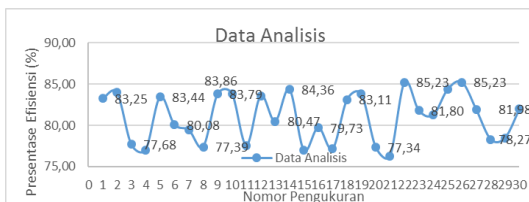
Gambar 17. Grafik Presentase (%) Efisiensi Trafo Inti Besi
