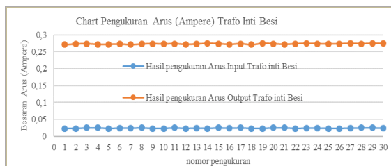
Gambar 14. Grafik Pengukuran Arus Trafo Inti Besi menggunakan beban baterai kering ( Lead Acid )
