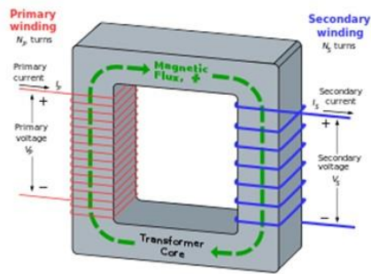
Gambar 2. Prinsip kerja Transformator
