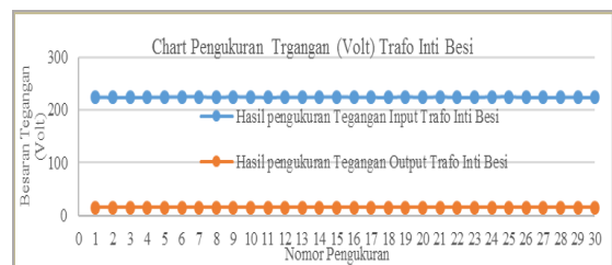
Gambar 13. Grafik Pengukuran Tegangan Trafo Inti Besi menggunakan beban baterai kering ( Lead Acid )
