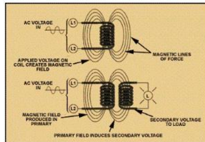
Gambar 1. Prinsip medan elektromagnetik
