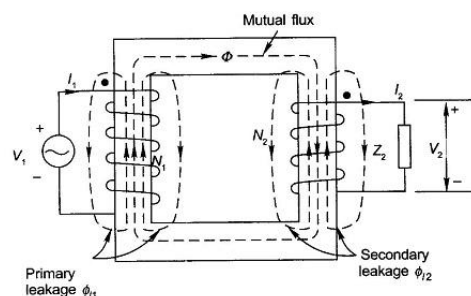
Gambar 3. Perbandingan antara fluks magnet dengan perbandingan tegangan dengan jumlah lilitan
