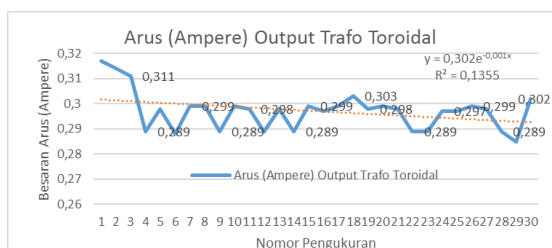
Gambar 20. Grafik Pengukuran Arus (Ampere) Pada Trafo Toroidal menggunakan beban baterai kering (Lead Acid)
