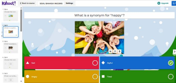
Gambar 1. Aplikasi Kahoot
